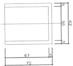
VISTA SUPERIOR Escala: 1/10
