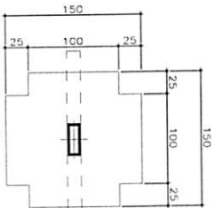
PLANTA Esc: 1/25
