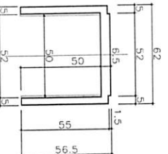
FRONTE Escala: 1/10
