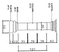
PIARES DO MURO Esc. 1/20
