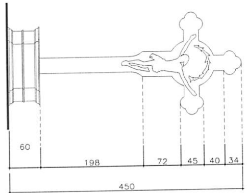
ELEVACÃO FRONTAL Esc: 1/25
