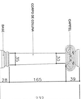
COLUNA Escala: 1/20
