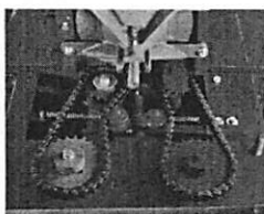
Caixa de engrenagens para mudança de tamanhos de corte, com parafuso de segurança de fácil remoção em caso de sobrecarga. Caja de engranajes para cambio de tamaños de corte, con perno de seguridad de sencilla reposición en situaciones de sobrecarga.
