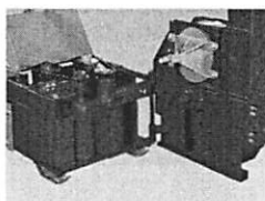
Sistema de alimentação com caixa articulável de 04 rolos e estrutura removível. Sistema de alimentación con caja articulable de 04 rollos y estructura removible.
