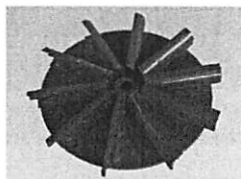
Rotor de disco 16mm aço carbono com 8, 10 e 12 facas em C, 4, 5 e 6 lançadores e sistema quebra grãos. Disco de corte opcional con 8, 10 y 12 cuchillas. 4, 5 y 6 lanzadores y sistema "quebra granos".
