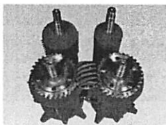
Sistema de transmissão com rosca sem fim (aço), e duas coroas de bronze lubrificadas em banho de óleo. Elimina a necessidade de lubrificação diária. Sistema de transmisión con sinfín de acero y dos engranajes de bronce lubricados en aceite. Elimina la necesidad de lubricación diaria.
